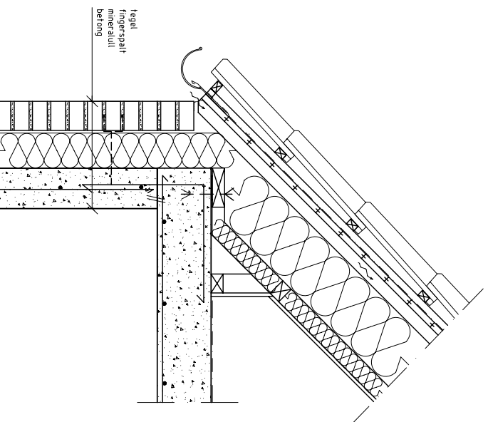
Detailj 49E Kombinationsvägg tegel/betong, ej utkragande takfot, betongbjälklag
