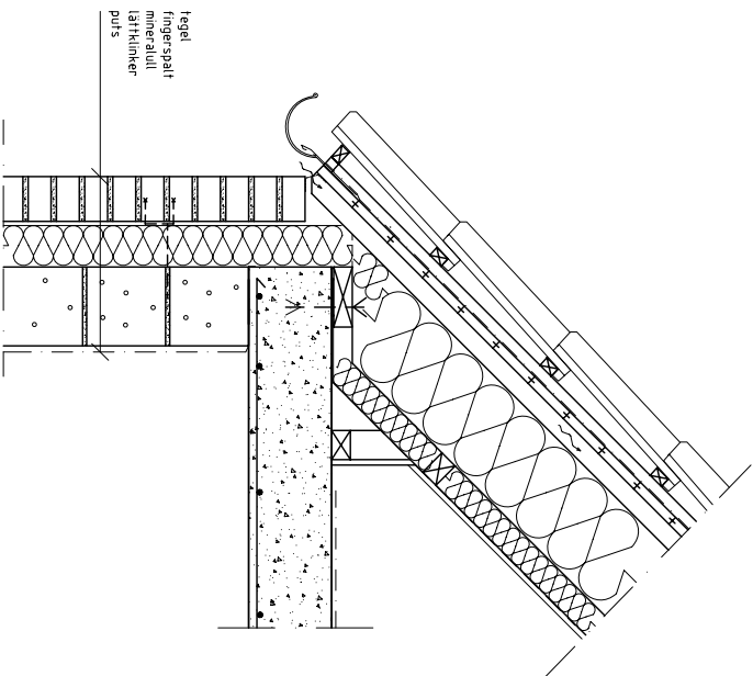
Detailj 49B Kombinationsmur tegel/lättklinker, ej utkragande takfot, betongbjälklag
