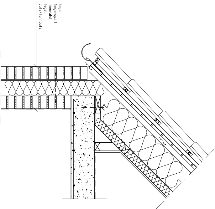
Detailj 49A Kanalmur tegel, ej utkragande takfot, betongbjälklag
