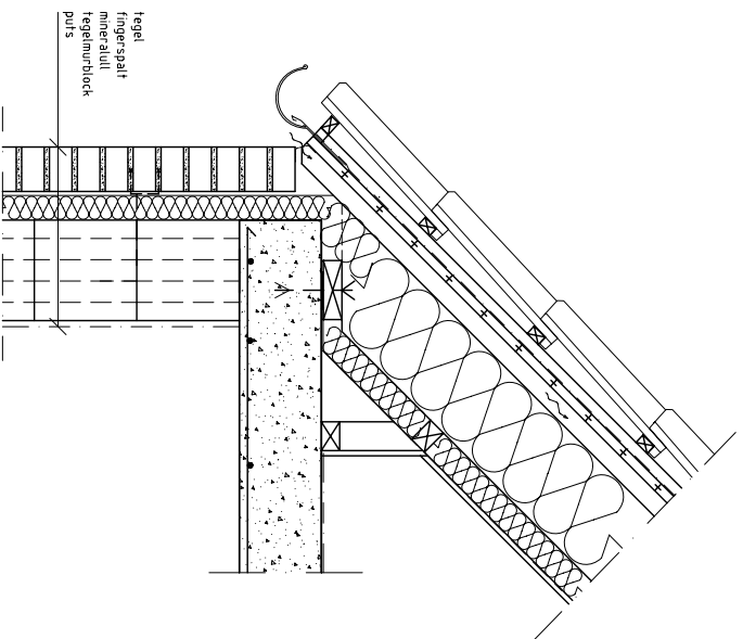
Detailj 49D Kombinationsmur tegel/tegelmurblock, ej utkragande takfot, betongbjälklag
