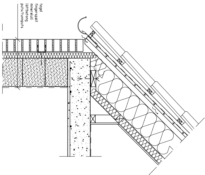
Detailj 49C Kombinationsmur tegel/lättbetong, ej utkragande takfot, betongbjälklag
