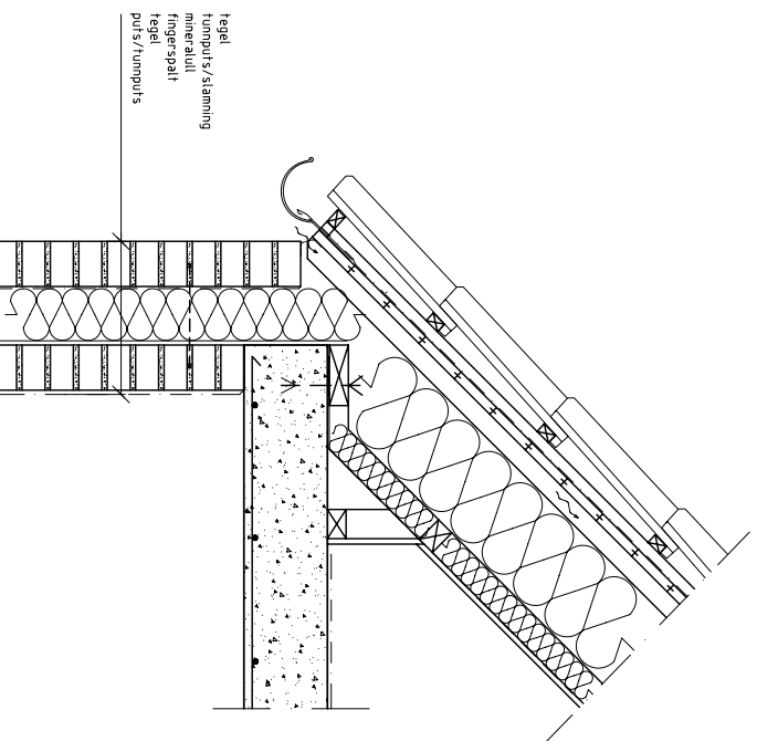
Detailj 50A Kanalmur tegel, fasadmurs insida slammad, betongbjälklag
